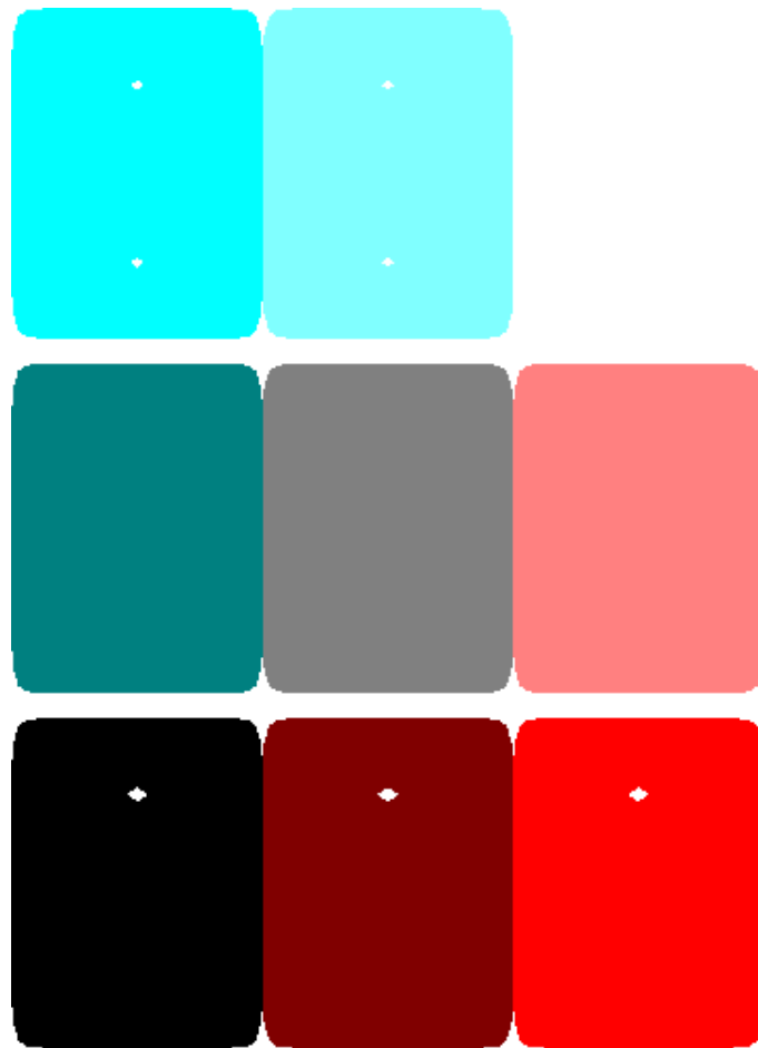
Abb. 11.1: Drittprojizierende Diagonalebene 1
