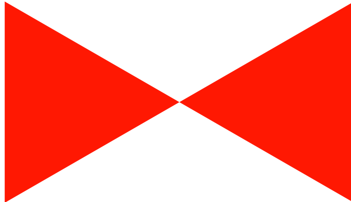
Abb. 0: Start mit zwei gleichseitigen Dreiecken
